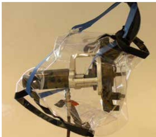
Exemple d'outil hydraulique avec protection et harnais
