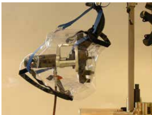
Esempio di attrezzo idraulico applicato con la protezione e la cinghia di arresto
